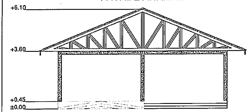
FACADE PRINCIPALE
