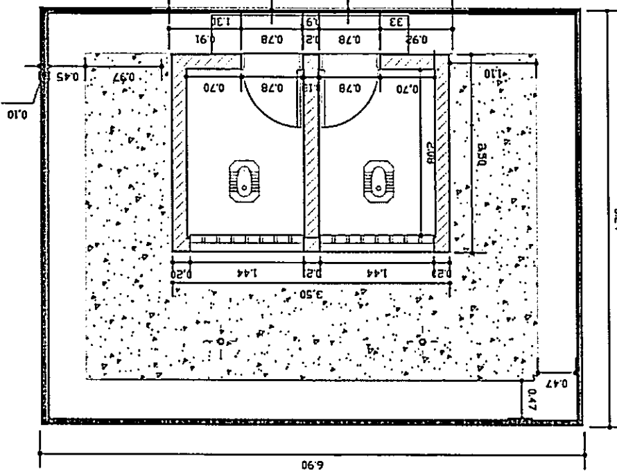
PLAN DE DISTRIBUTION TOILETTE
